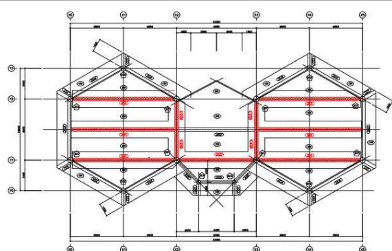
부재보강 위치도
