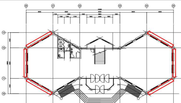
내진보강 위치도
